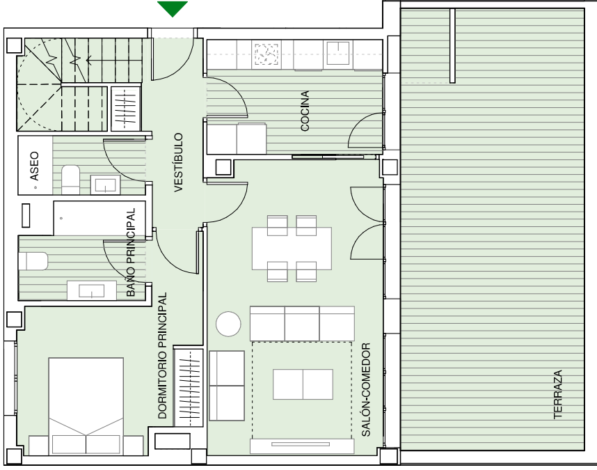
PLANTA BAJA
